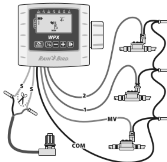
PODŁĄCZENIE ZAWORÓW
